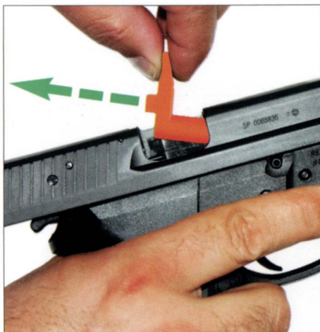
1 - Retrait du témoin de chambre vide
