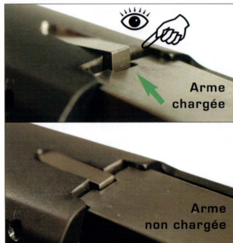
4 - Contrôle du chargement
