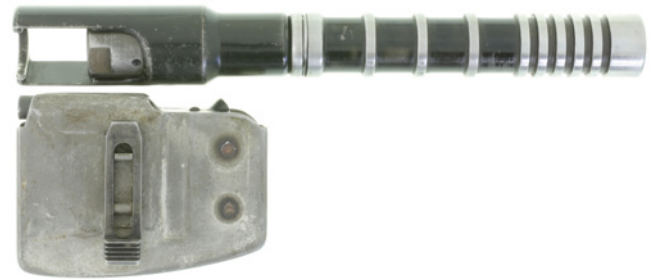
59901 CHF 150.- 282381 Schiessbecher für Panzerwurfgranate zu K31, 7.5x55. TL 210 mm, Ganzstahl, schwarz Syncorite beschichtet. Hier handelt es sich um die zweite Ausführung mit gefederter Halterung. Promatverzinktes Treibpatronenmagazin zu K31. #ohne SON Zustand 1
